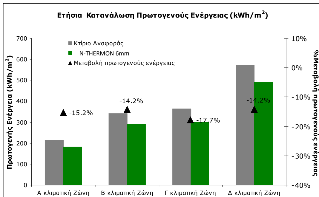
Σχήμα 2 Ετήσια κατανάλωση πρωτογενούς ενέργειας για τη μονοκατοικία πριν (κτίριο αναφοράς) και μετά (N-THERMON 6mm) την εφαρμογή προϊόντων της NEOTEX ΑΕΒΕ.
